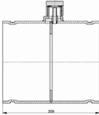
Ölçüler / Dimensions (mm)
